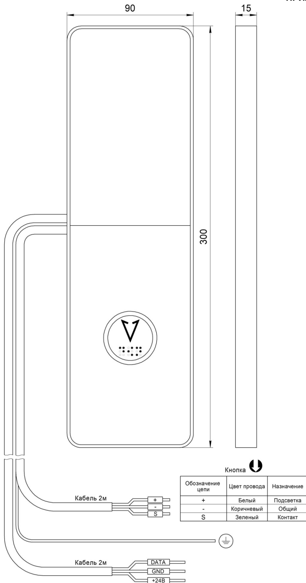
Рис.1 Внешний вид Вызывной пост ОНИКС НШЕК.468381.027-01
